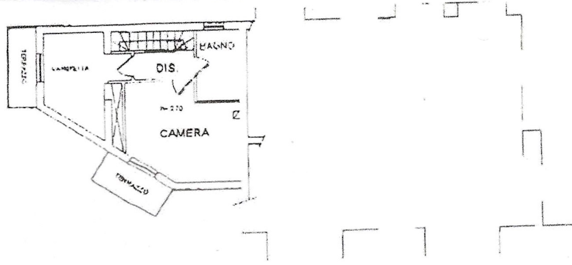
PIANO PRIMO
